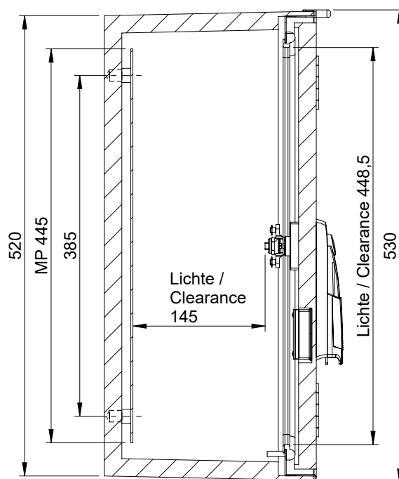
B-B
